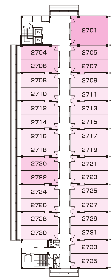
7階平面図
